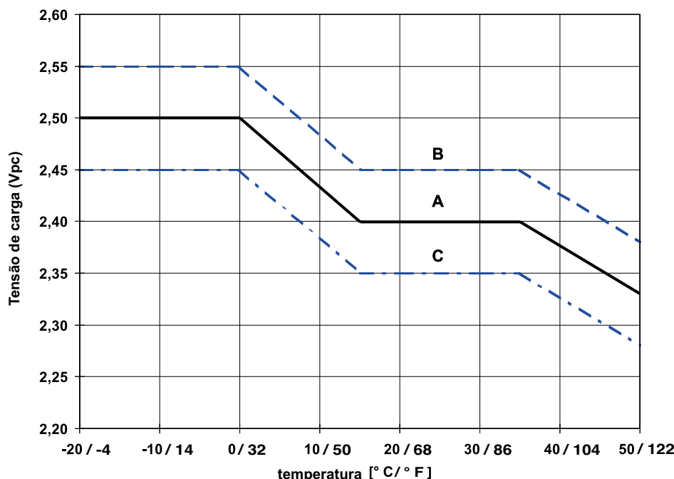
Fig. 1: Tensão de carga vs. temperatura para modo solar. Modos de carga:
