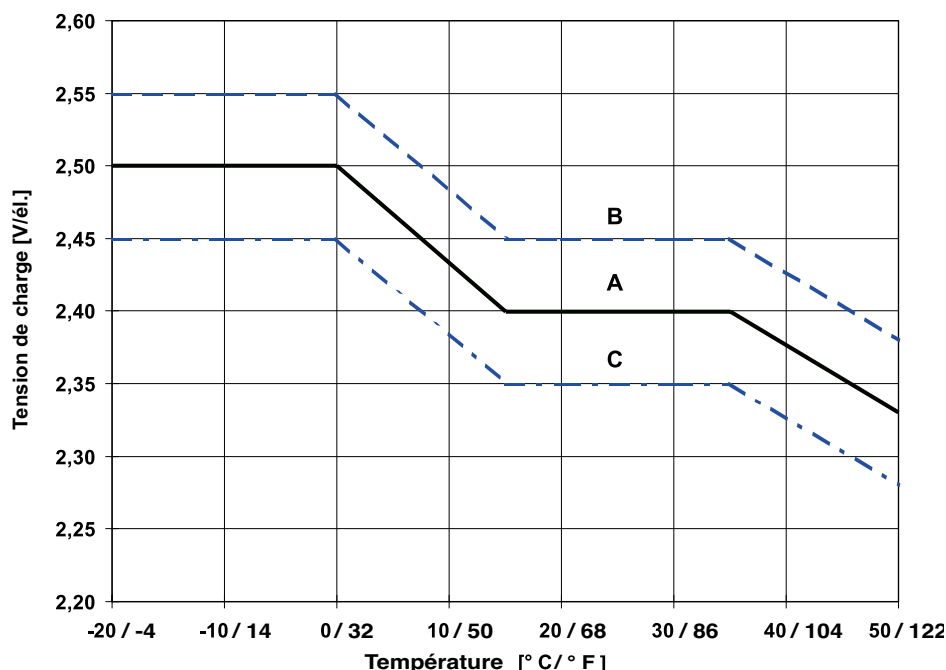
Fig. 1: Tension de charge selon les températures pour un service solaire.
