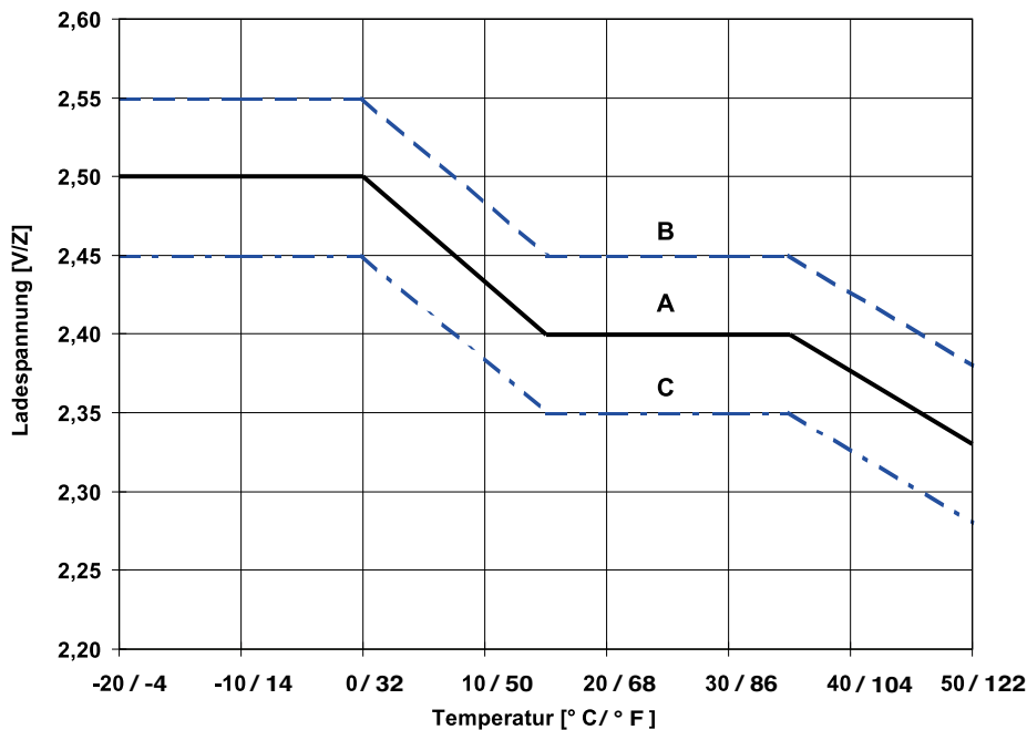
Bild 1: Ladespannung über Temperatur für Solar-Betrieb. Ladearten:
