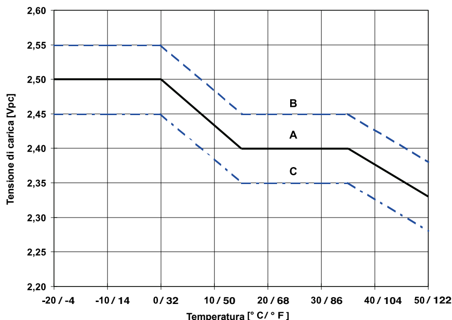
Figura 1: tensione di carica per temperatura – Modalità Solar. Metodi di carica:
