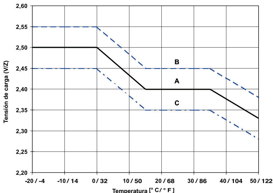
Figura 1: Tensión de carga respecto de la temperatura para el funcionamiento solar.
